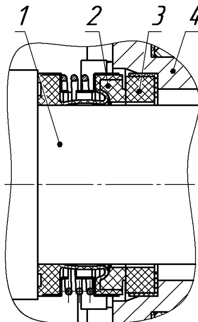
Рисунок 2 – Уплотнение торцовое
