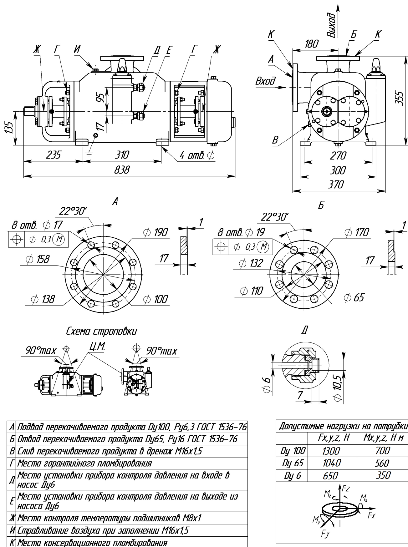
Рисунок Б3 Габаритный чертеж насоса типа А2 2ВВ10/16, А2 2ВВ 16/16, А2 2ВВ 25/16
